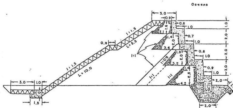
Fig. 35 Muro de defensa contra tsunamis en Taro
