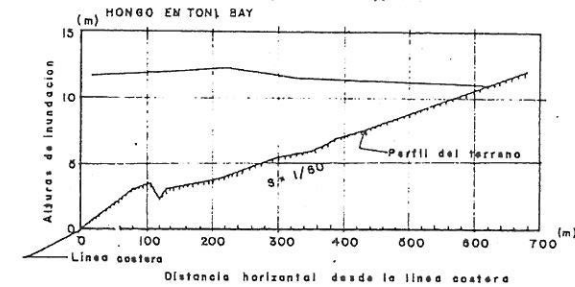
fig. 9 Traza de la línea de inundación en Hongo Toni bay, Japon
