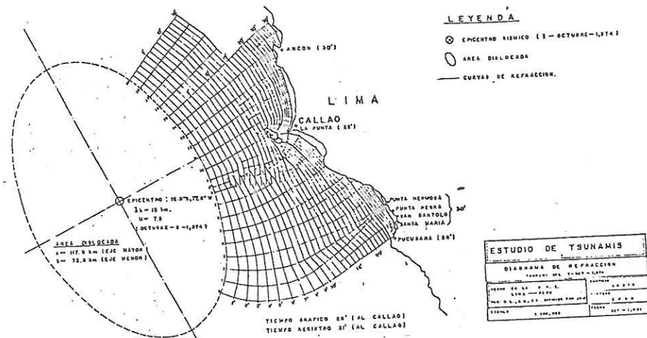
Fig. 18 DIAGRAMA DE REFRACCIÓN DEL TSUNAMI DEL 3 DE OCTUBRE DE 1974.
