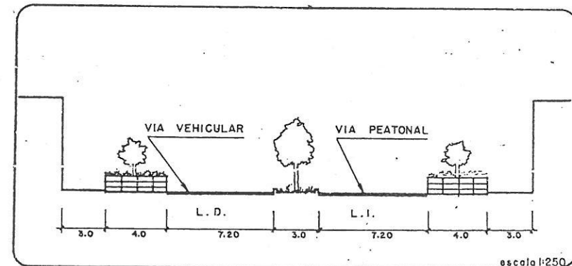
fig.30b. Corte transversal de la Av. Guardia Chalaca
