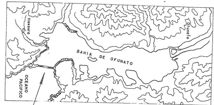
Fig. 33 UBICACION DEL ROMPEOLAS EN LA BAHIA DE OFUNATO
