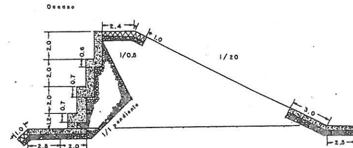
Fig. 36 Muro de defensa contra Tsunami en Yoshihama
