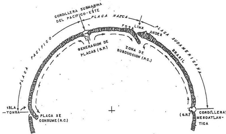
Fig. 3. CORTE ESQUEMÁTICO DEL GLOBO TERRAQUEO Se observa la Placa Nazca, la Placa Sudamericana y la Placa Pacífico. (CORTE A-A DE LA Fig. 2).
