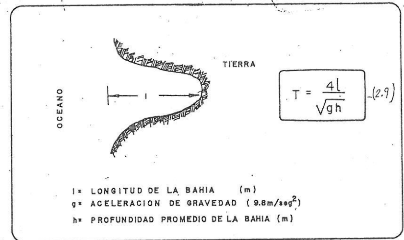
fig. 8 Cálculo del período de una bahía
