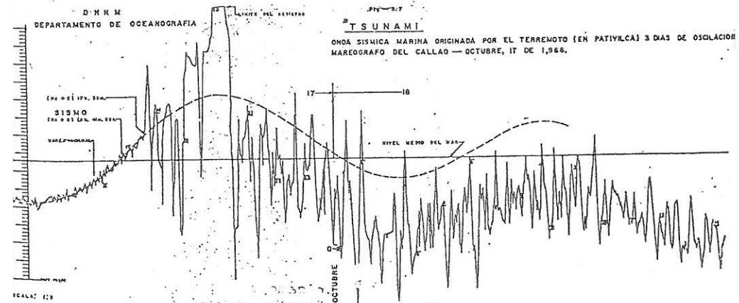
Fig. 17 REGISTRO DEL TSUNAMI DEL 17 / 1966 OBTENIDO EN EL MAREOGRAFO DE LA PUNTA - CALLAO (CORTESIA DE LA DIRECCION DE HIDROGRAFIA Y NAVEGACION DE LA MARINA DE GUERRA DEL PERU)
