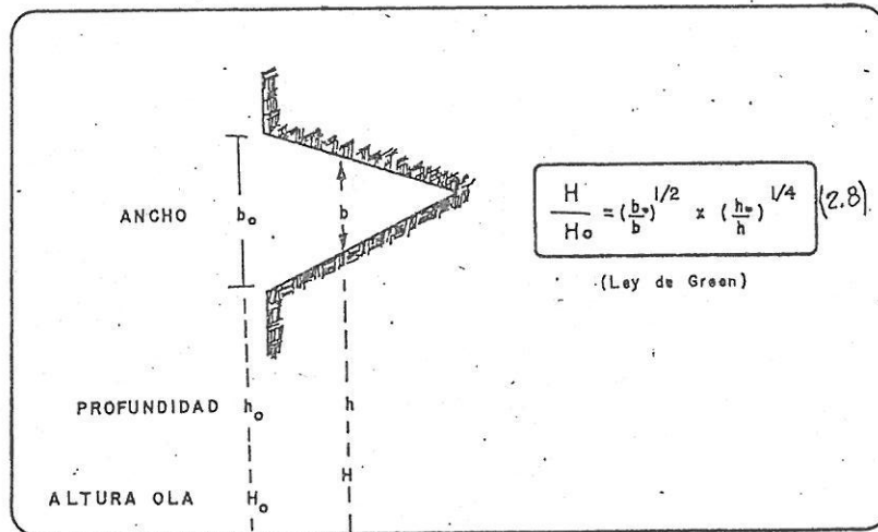
Fig. 7 Influencia de la configuración geométrica de la bahía sobre la altura de ola
