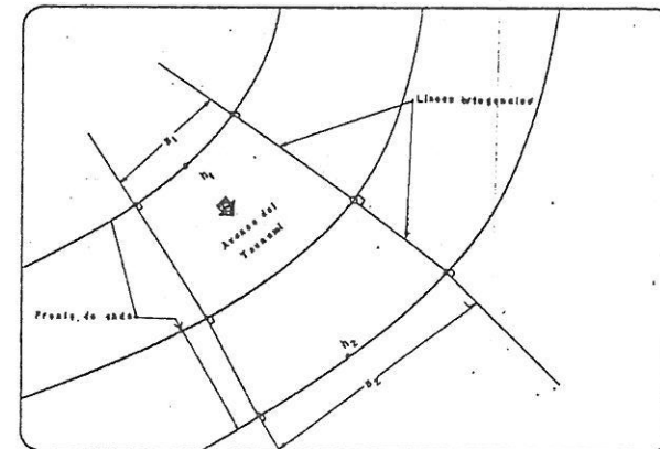
FIG. N° 4 LEY DE GREEN
