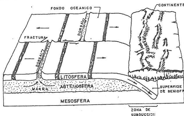
Fig. 1 ISOMETRICO DE DORSALES, ZONAS DE FRACTURA Y DE SUBDUCCION
