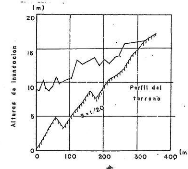
fig. 11 Traza de la línea de inundación en Sasu Toni bay Japon
