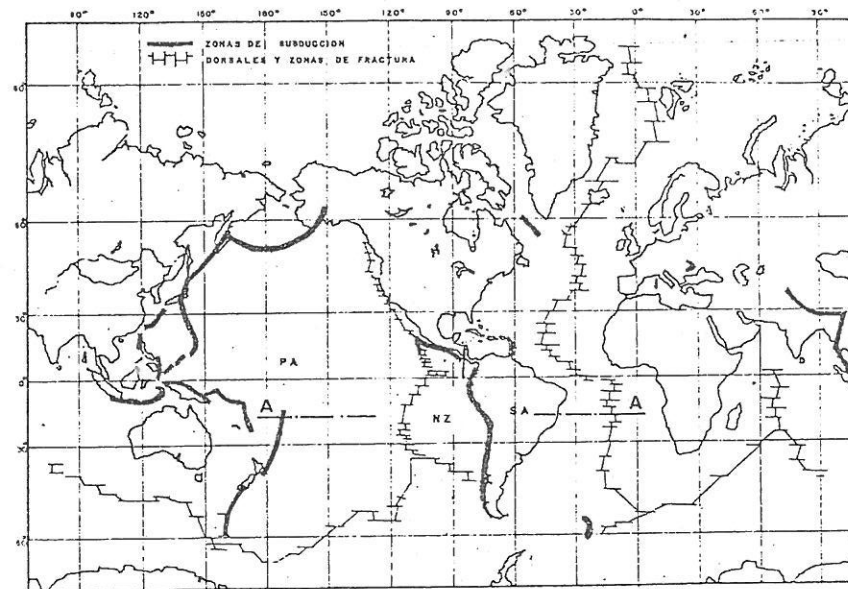
Fig. 2 Teoría de placas. SA=Placa Sudamericana, PA=Placa Pacífica, NZ=Placa Nazca, A=Placa Australiana, I=Placa Indiana, U=Placa Uraliana, E=Placa Euroasiática, A=Placa Africana, A=Placa Antártica, C=Placa Cocos.
