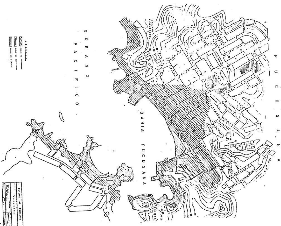
Fig. 23 AREAS INUNDABLES Y ZONAS DE REFUGIO EN PUCUSANA.
