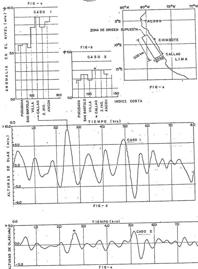
REGISTRO SIMULADO FRENTE A LIMA A 20mts. DE PROFUNDIDAD 1- LEVANTAMIENTO UNIFORME 2- LEVANTAMIENTO VARIABLE
