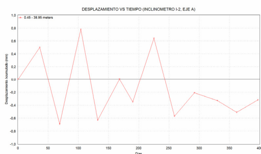
Figura 10. Gráfico de desplazamiento vs tiempo obtenido de medición inclinométrica
