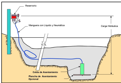
Figura 6. Detalle de instalación de celda de asentamiento
