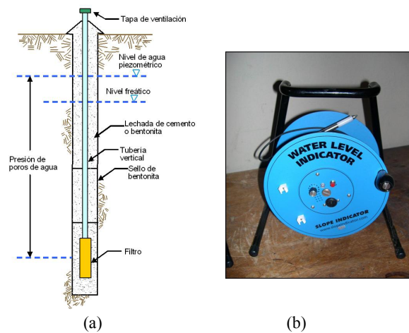
Figura 4. (a) Instalación de piezómetro eléctrico de tipo Casagrande (b) Indicador de nivel de agua
