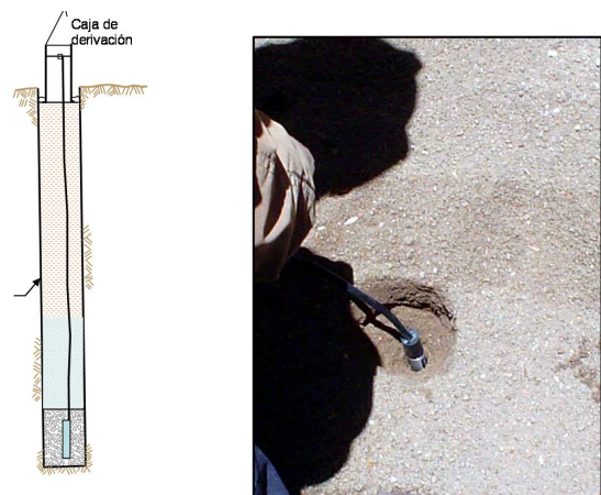
Figura 5. Instalación de piezómetro eléctrico de cuerda vibrante
