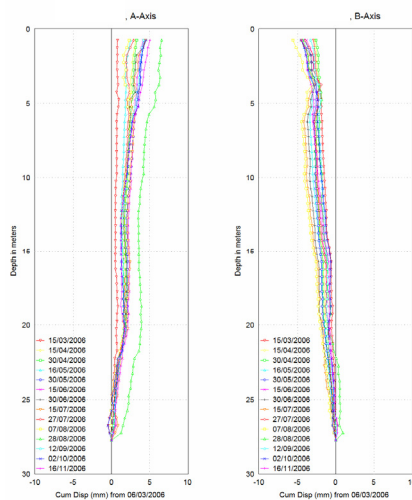
Figura 9. Gráfico de desplazamientos acumulados obtenido de medición inclinométrica
