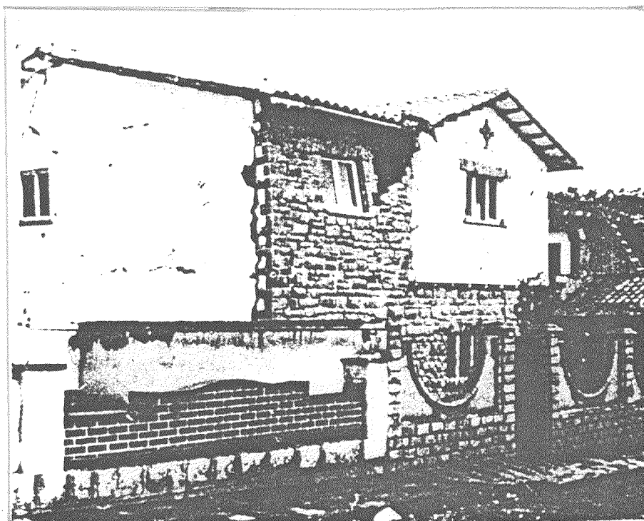
Foto No. 10.— Agrietamientos en paredes de casa, después del terremoto del Cuzco, el 21 de Mayo de 1950.
